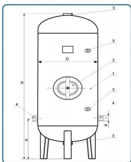
Budowa zbiornika hydroforowego: 1 - zbiornik, 2 - wyczystka, 3 - króciec 2", 4 - króciec wlotowo-wyjłowy, 5 - króciec wodowskazu 1/2"
