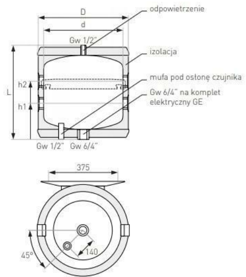
4.1. Schemat zbiorników buforowych SG(B) 40, 60, 80, 100, 120, 140 wiszących, bez węzownicy
