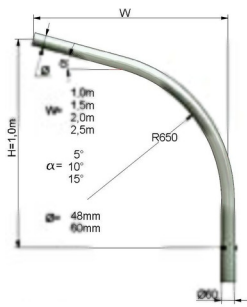
Wysięgnik NT ST-Y/1rW= / \alpha = / \emptyset =
