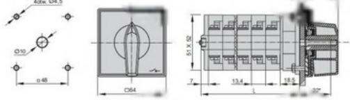
Wymiary. Łączniki ŁK16R, 25R, 32R o liczbie segmentów n=1..10
