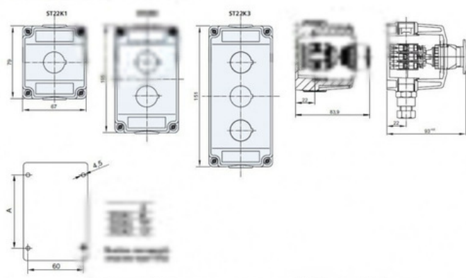
Wymiary kaset ST22K1 i ST22K3
